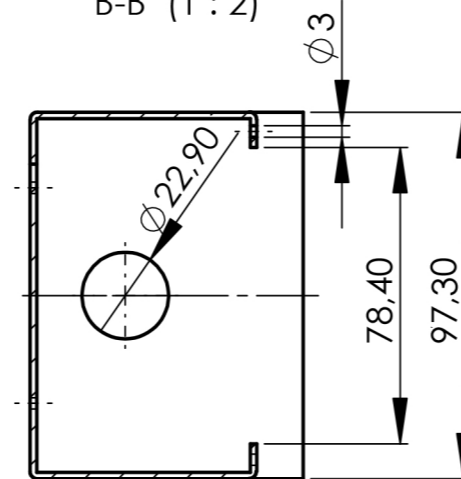
B-B (1:2)
