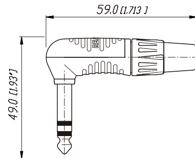
RP3RC
