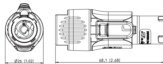
RCAC31-G / RCAC30-G
