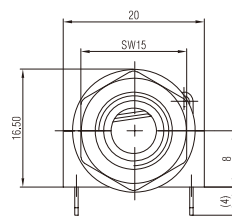
NYS212
