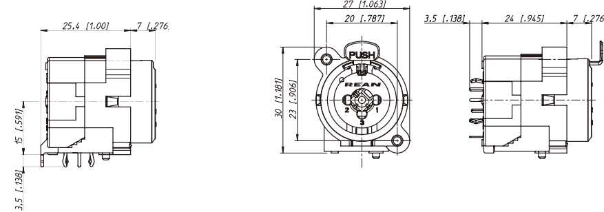
RCJ9FI-V
